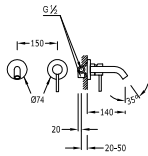
Monomando a muro Single lever wall washbasin mixer Jednopáková nástěnná baterie
