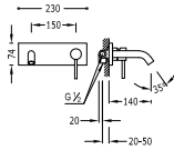
Monomando a muro Single lever wall washbasin mixer Jednopáková nástěnná baterie
