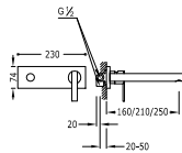
Monomando a muro LEX-TRES Single lever wall mixer LEX-TRES Jednopáková nástěnná baterie LEX-TRES
