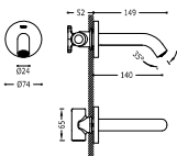
Canna parete Wall spout Nástěnné ramínko
