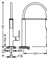
Monocomando lavello verticale CUADRO estraibile Single lever single hole sink mixer CUADRO with removable spout Jednopaková dřezová kuchyňská baterie CUADRO s vyjímatelným kropicítkem
