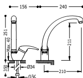
Monocomandoavello verticale BASIC Single lever single hole sink mixer BASIC Jednopáková dřezová kuchyňská baterie BASIC
