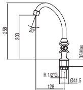
Rubinetto laterale Lateral tap Baterie s bočním ovládním
