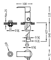
Monocomando bidet con doccia Bidet mixer tap with small shower head Jednopáková bidetová baterie se sprškou
