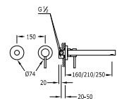
Monomando a muro MAX-TRES Single lever wall washbasin mixer MAX-TRES Jednopáková nástěnná baterie MAX-TRES
