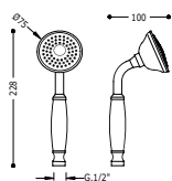
Doccetta anticalcare RETRO Antilime shower RETRO Sprcha, proti usaz. vod. kamene RETRO
