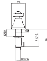
Rubinetto laterale Lateral tap Boční umyvadlová baterie
