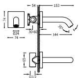
Canna parete Wall spout Nástěnné ramínko
