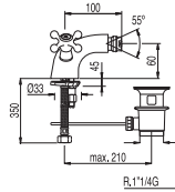
Monoblocco bidet Single hole bidet mixer Dvoupáková bidetová baterie
