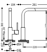
Monocomando lavello verticale CUADRO estraibile Single lever single hole sink mixer CUADRO with removable spout Jednopaková dřezová kuchyňská baterie CUADRO s vyjímatelným kropicítkem
