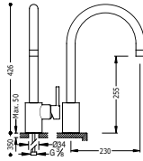
Monocomando lavello verticale MAX Single lever single hole sink mixer MAX Jednopaková dřezová kuchyňská baterie MAX
