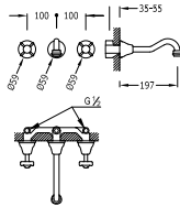
Accumulatore lavabo a muro Wash-basin mixer Nástěnná umyvadlová baterie
