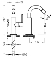
Monocomando bidet Single lever bidet mixer Jednopáková bidetová baterie
