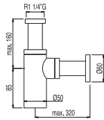
Sifone telescopico a vista per lavabo Telescopic visible basin drain trap Výsuvný umyvadlový viditeľný sifon
