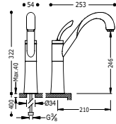
Monocomandoavello verticale Single lever single hole sink mixer Jednopaková dřezová baterie svislá
