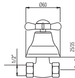
Rubinetto di arresto filettato 1/2" Valve 1/2" Uzavírací ventil 1/2"
