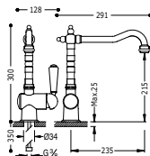
Monocomandoavello verticale RETRO-TRES Single lever single hole sink mixer RETRO-TRES Jednopáková dřezová kuchyňská baterie RETRO-TRES
