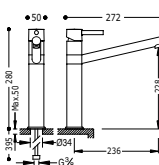
Monocomando lavello verticale ALPLUS canna lunga Single lever single hole sink mixer ALPLUS tube spout Jednopáková dřezová kuchyňská baterie ALPLUS dlouhé ramínko
