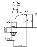
Rubinetto lavandino 1 acqua o premiscelata 1 water or premixed bathroom tap Umyvadlová baterie pro jednu nebo předem smíchanou vodu
