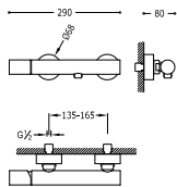
Monocomando doccia Doccetta anticalcare (034.116.01) con supporto orientabile. Flessibile satin (91.34.609.15).
