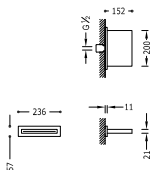
Bocca a cascata set doccia Cascade cast spout bath mixer Ramínko s vodopádem k baterii pro vanu-sprchu nebo umyvadlo
