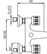
Gruppo vasca Doccetta anticalcare con supporto orientabile. Flessibile doppia graffatura
