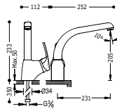
Monocomando lavello verticale Single lever single hole sink mixer Jednopláková dřezová baterie svislá
