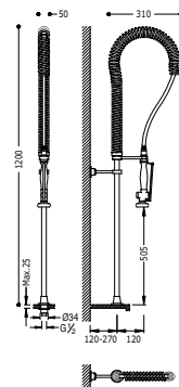
Monocomando lavello verticale Single lever single hole sink mixer Dřezová kuchyňská baterie
