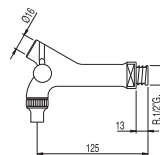
Rubinetto vino N° 2/N Wine tap N° 2/N Kohoutek na víno č. 2/N
