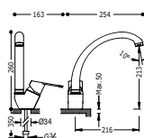
Monocomandoavello verticale BM-TRES Single lever single hole sink mixer BM-TRES Jednopáková dřezová kuchyňská baterie BM-TRES
