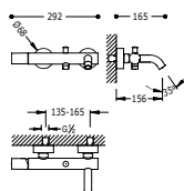
Monocomando vasca Doccetta anticalcare con supporto orientabile. Flessibile satin (91.34.609).
