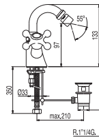
Monoblocco bidet Single hole bidet mixer Dvoupáková bidetová baterie
