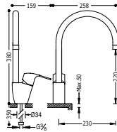
Monocomando lavello verticale K-TRES Single lever single hole sink mixer K-TRES Jednopáková dřezová kuchyňská baterie K-TRES
