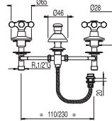
Accumulatore bidet con doccetta Single hole bidet mixer with small shower head Bidetová baterie se sprškou
