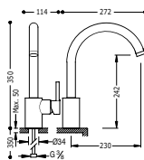
Monocomando lavello verticale MAX-TRES Single lever single hole sink mixer MAX-TRES Jednopáková dřezová kuchyňská baterie MAX-TRES
