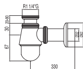
Sifone a bottiglia facilmente ispezionabile per bidet Self-inspecting bottle-type drain trap for bidet Bidetový lahvový sifon, rozšroubovateľný
