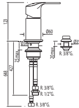
Monocomando bidet con doccia Bidet mixer tap with small shower head Jednopáková bidetová baterie se sprškou
