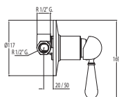
Monocomando incasso (1 via) corpo incassato incluso Built-in mixer taps (1 way) Built-in body included Vestavěná jednopáková baterie (jednocestný) včetně podomítkového tělesa
