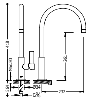
Monocomando lavello verticale CLASS-TRES Single lever single hole sink mixer CLASS-TRES Jednopáková dřezová kuchyňská baterie CLASS-TRES
