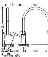
Monocomando lavello verticale ALPLUS Single lever single hole sink mixer ALPLUS Jednopáková dřezová kuchyňská baterie ALPLUS
