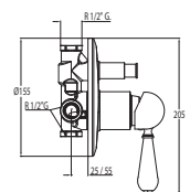
Monocomando incasso (2 vie) corpo incassato incluso Built-in mixer taps (2 way) Built-in body included Vestavěná jednopáková baterie (dvoucestný) včetně podomítkového tělesa
