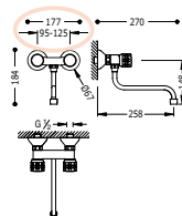
Gruppo lavello parete Distanza da parete di 260 mm. Wall sink mixer Distance from wall 260 mm. Nástěnný dřezový celek vzdálenost od zdi 260 mm
