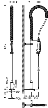
Monocomando lavello verticale Single lever single hole sink mixer Jednopáková dřezová kuchyňská baterie
