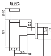
Sifone telescopico a vista per lavabo Telescopic visible basin drain trap Čtverhranný, výsuvný umyvadlový sifon viditeľný
