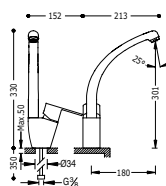
Monocomando lavello verticale BM-TRES Single lever single hole sink mixer BM-TRES Jednopáková dřezová kuchyňská baterie BM-TRES
