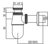
Sifone a bottiglia facilmente ispezionabile per lavabo Self-inspecting bottle-type drain trap for basin Umyvadlový lahvový sifon, rozšroubovateľný
