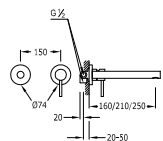
Monomando a muro MAX Single lever wall washbasin mixer MAX Jednopáková nástěnná baterie MAX
