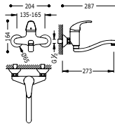
Monocomando a muro Single lever wall sink mixer Jednopáková dřezová baterie nástěnná
