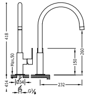
Monocomando lavello verticale LOFT-TRES Single lever single hole sink mixer LOFT-TRES Jednopáková dřezová kuchyňská baterie LOFT-TRES
