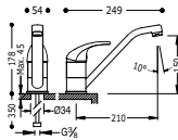
Monocomando lavello verticale * (per modelli anteriori al listino 2007 ... 91.34.290) Single lever single hole sink mixer * (for models before price list 2007 ... 91.34.290) Jednopáková dřezová baterie svislá * (do roku 2007 ... 91.34.290)
